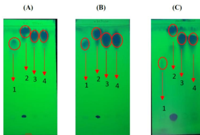
Gambar 1. Hasil Hasil Kromatografi Lapis Tipis dengan Fase Gerak Etil Asetat : Etanol ( 2 : 1 v/v ) (A), n-heksana : Etanol ( 2 : 1 v/v ) (B) dan Kloroform : Etanol ( 4 : 1 v/v ) (C) (Keterangan : 1. Asam Salisilat; 2. 4-klorometil benzoi klorida; 3. Asam 4-(klorometil)salisilat; 4. Asam 4-(klorometil)salisilat terdahulu)
