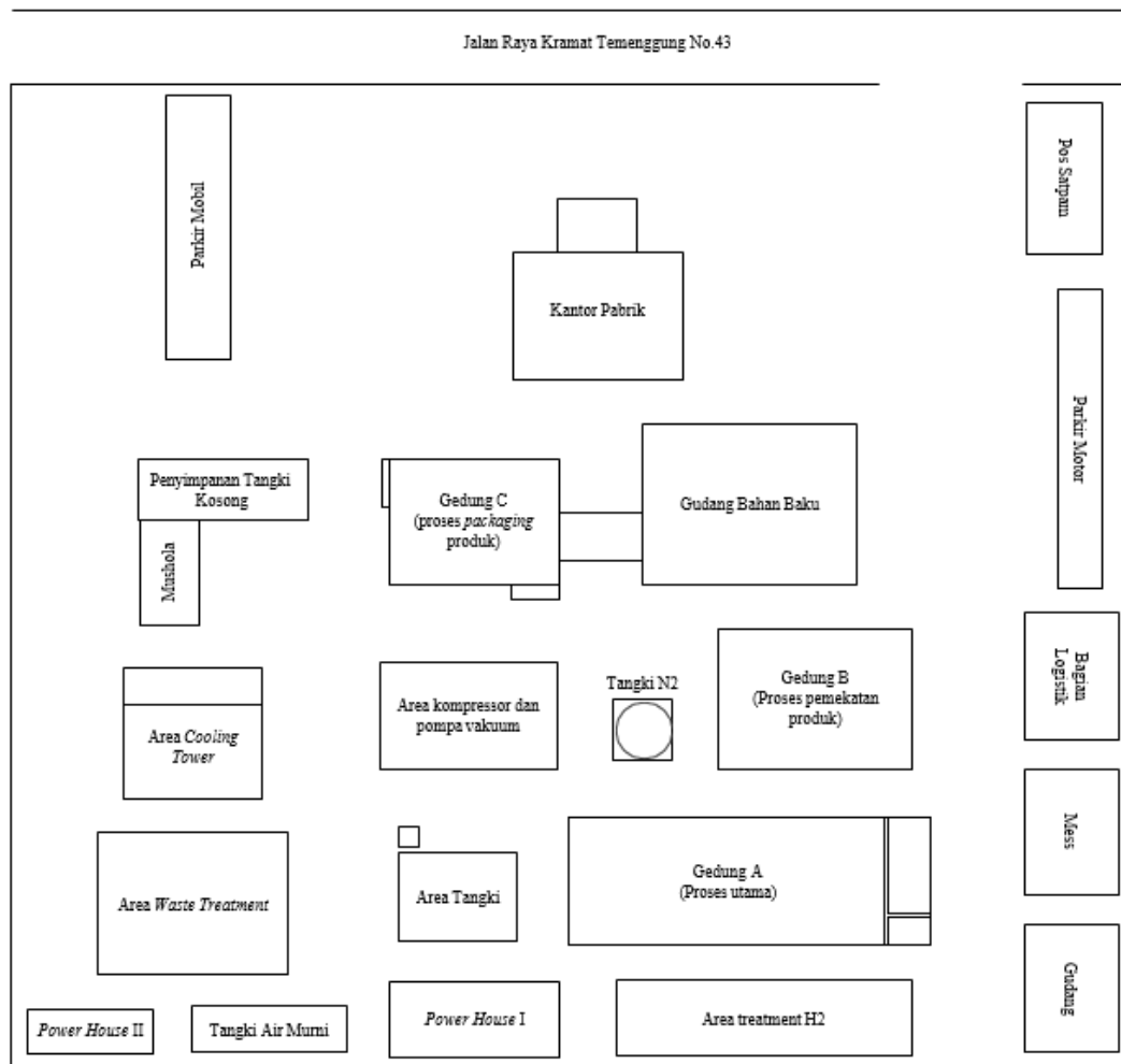
Gambar I.2. Tata Letak Pabrik PT Sindopex Perotama
