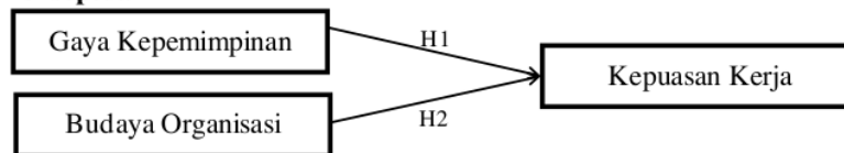
Gambar 1 Kerangka Pemikiran
