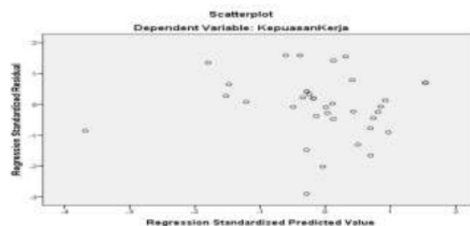
Gambar 2 Grafik Scatterplot
