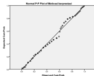
Gambar 2 : Normal P Plot Motivasi Berprestasi
