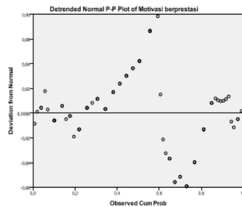
Gambar 5 : Diagram pencar Motivasi Berprestasi
