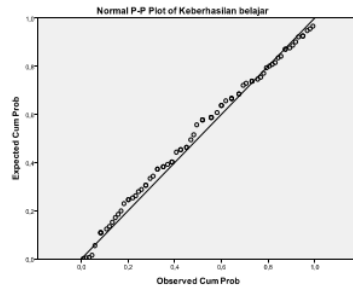
Gambar 4 : Normal P Plot Keberhasilan Belajar
