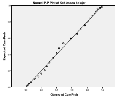
Gambar 3 : Normal P Plot Kebiasaan Belajar
