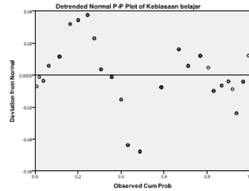
Gambar 6 : Diagram pencar Kebiasaan Belajar
