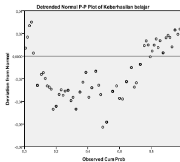
Gambar 7 : Diagram pencar Keberhasilan Belajar
