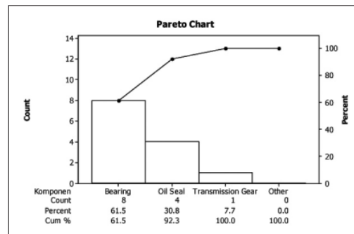
Gambar 3. Analisis pareto dari reaktor kimia nomer 1
