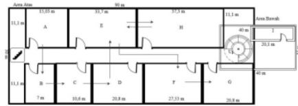
Gambar 3. Lay-out Usulan
