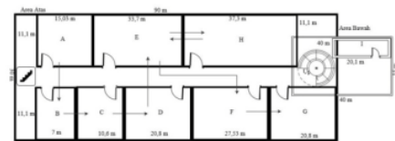
Gambar 5.2. Lay-out usulan
