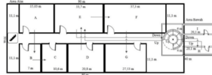
Gambar 4.1. Layout Awal
