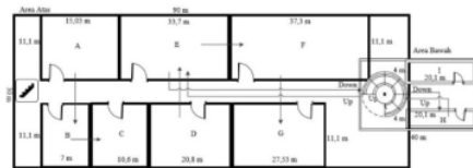
Gambar 5.1. Lay-out awal
