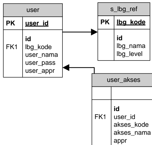
Gambar 5. ERD User dan Hak Akses
