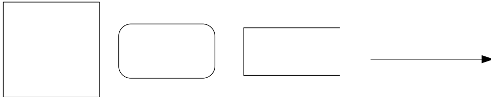
Gambar 2. Bentuk DFD
