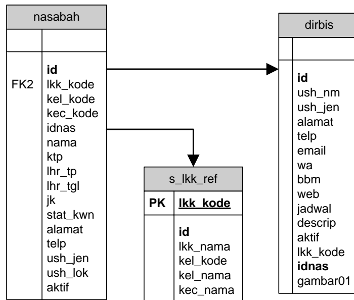
Gambar 6. ERD Nasabah dan Informasi Bisnis
