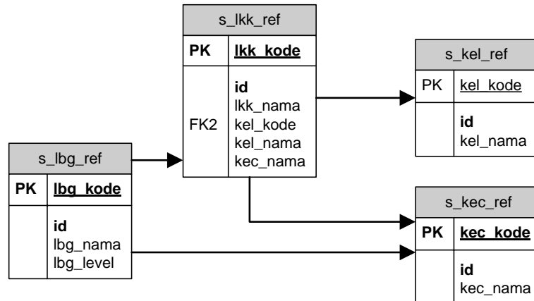
Gambar 4. ERD Kelembagaan
