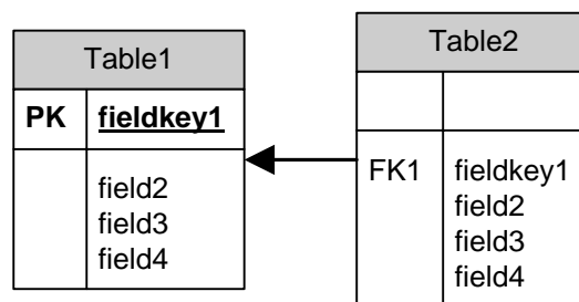
Gambar 1. Bentuk ERD
