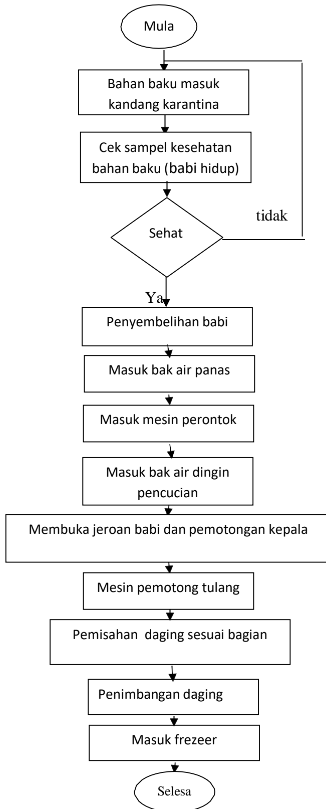
Gambar 2.3 : Diagram alir proses produksi
