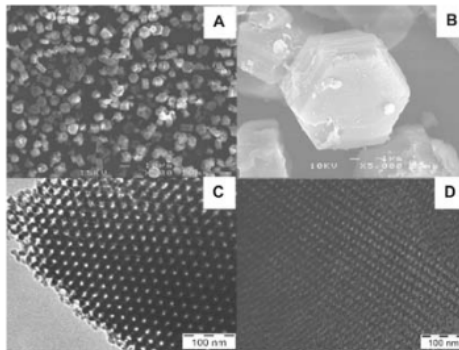
Gambar 1. Gambar scanning electron microscope (SEM) dari FDU-12 (A,B) dan gambar dari Transmission Electron Microscope (TEM) dari FDU-12 yang termodifikasi (C,D) (Sandy Budi Hartono, 2009).
