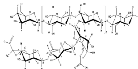
Gambar 1 Struktur kimia xanthan gum (Anonim,2005)
