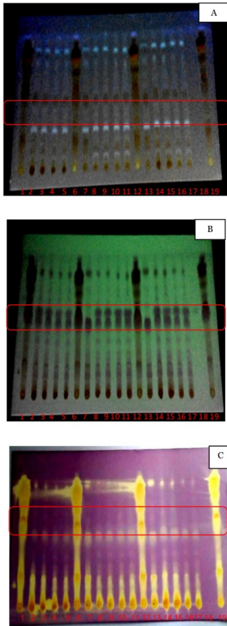
GAMBAR 2. Profil zat aktif berkhasiat (alfa mangosteen) dibawah sinar UV 254 nm tanpa penampak noda (A), sinar UV 366 nm (B) dan setelah penyemprotan dengan DPPH (C) Terdapat 19 noda, dimulai dari kiri: pembanding (isolat) (1), formula A (2),(3), formula B (4),(5), isolat (6), ekstrak kering (7), formula C (8),(9), formula D (10),(11), isolat (12), ekstrak kering (13), formula A (14), formula B (15), formula C (16), formula D (17), formula blangko (18), isolat alfa mangosteen (19).
