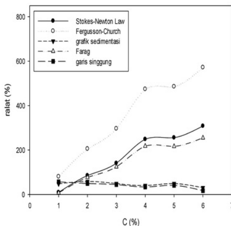
Gambar 9. Hubungan antara Konsentrasi (C) vs Ralat pada Diameter Tabung = 8 cm
