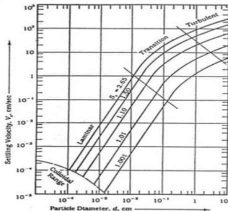
Gambar 4. Grafik Kecepatan Sedimentasi [8]
