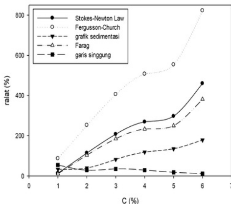
Gambar 11. Hubungan antara Konsentrasi (C) vs Ralat pada Diameter Tabung = 10,5 cm
