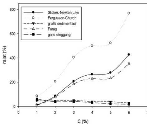
Gambar 10. Hubungan antara Konsentrasi (C) vs Ralat pada Diameter Tabung = 8,5 cm
