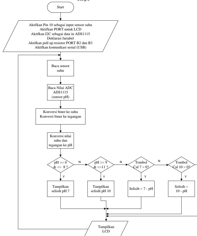
Gambar 8. Diagram alir perangkat lunak
