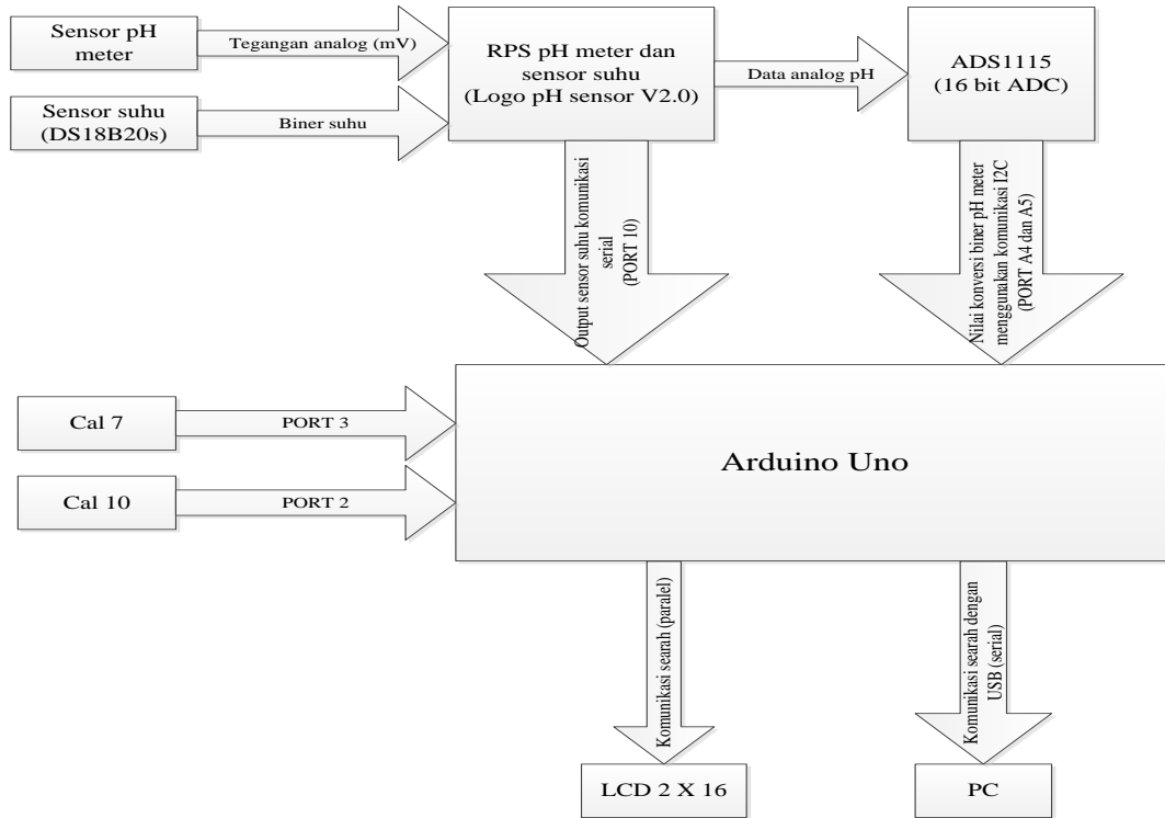
Gambar 4. Diagram blok alat
