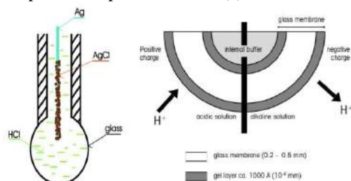
Gambar 1. Sensor pH: a) konstruksi, b) ilustrasi proses pengukuran pH (Sumber: Vanysek, 2004, diakses pada 20 Juni 2017)
