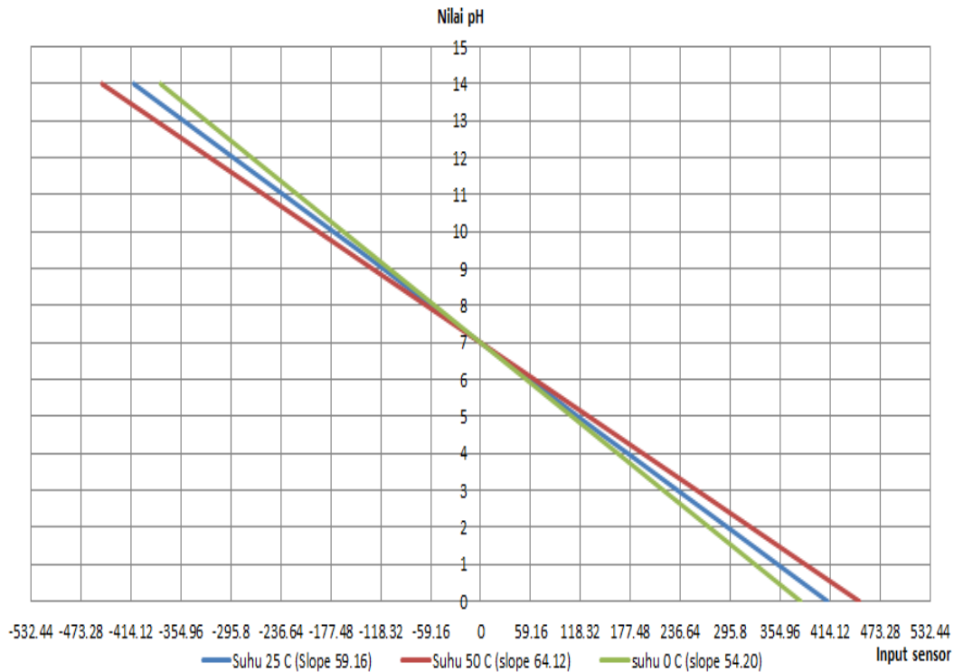
Gambar 2. Kurva beda potensial sensor terhadap pH terukur yang dipengaruhi suhu (Sumber: Vanysek, 2004, diakses pada 20 Juni 2017)
