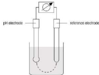
Gambar 3. Ilustrasi cara pengukuran pH larutan (Sumber: Vanysek, 2004, diakses pada 20 Juni 2017)
