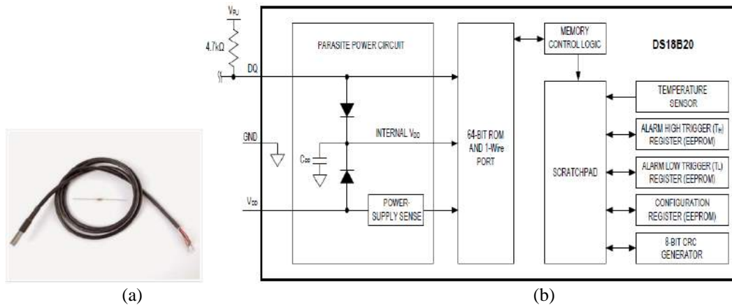
Gambar 7. Modul sensor suhu DS18B20s, a) bentuk fisik, b) diagram blok (Sumber: Maxim integrated products, Inc, 2015, diakses pada 20 Juni 2017)
