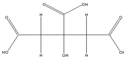
Gambar 2.2. Struktur Kimia Asam Sitrat Sumber: Hasibuan (2010)
