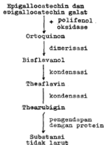
Gambar 5.4. Skema Pembentukan Theaflavin dan Thearubigin Sumber : Harler, 1963
