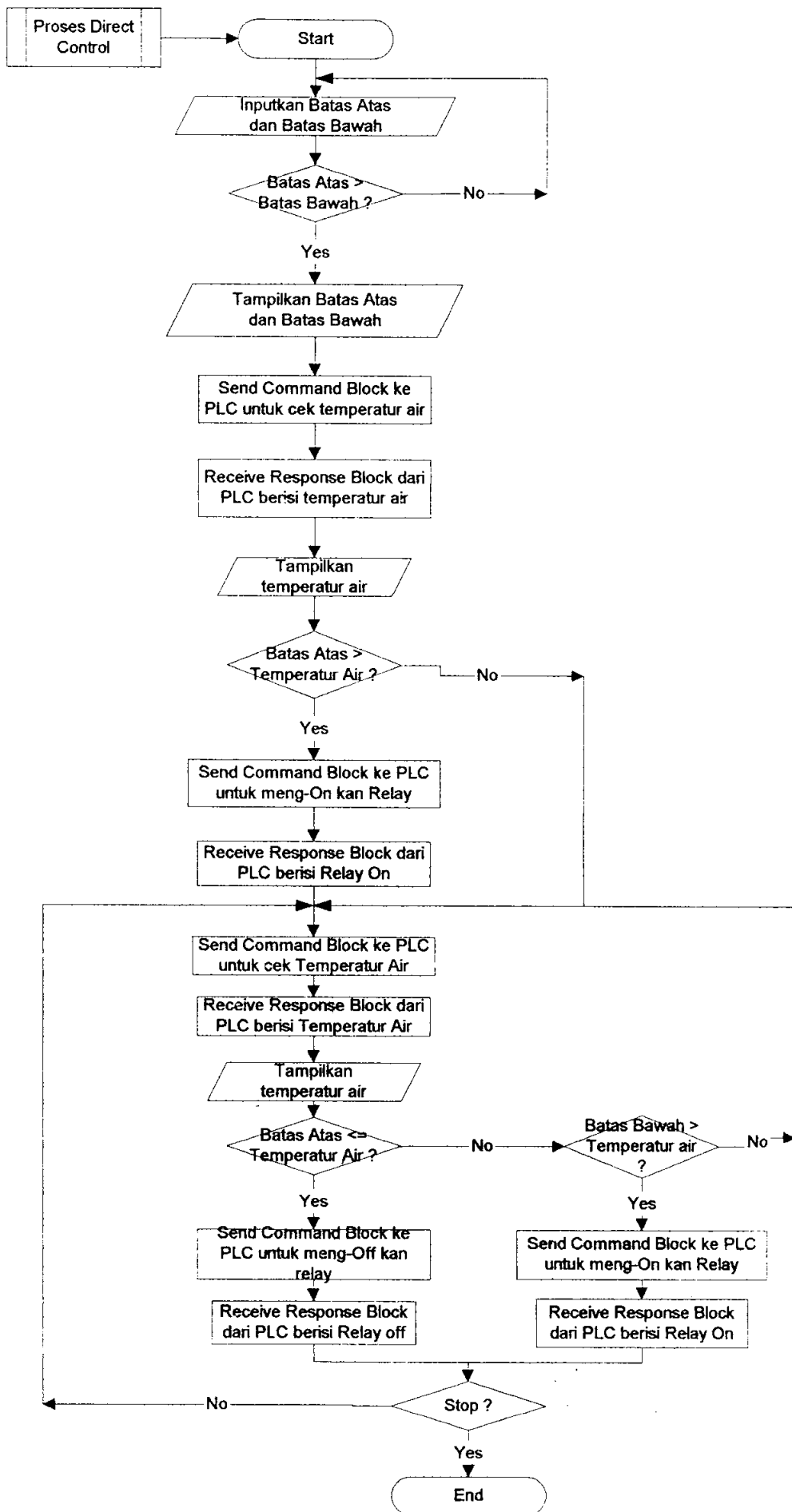
GAMBAR L-2 GAMBAR DIAGRAM ALUR MENU APLIKASI (DIRECT CONTROL) KOMPUTER -PLC
