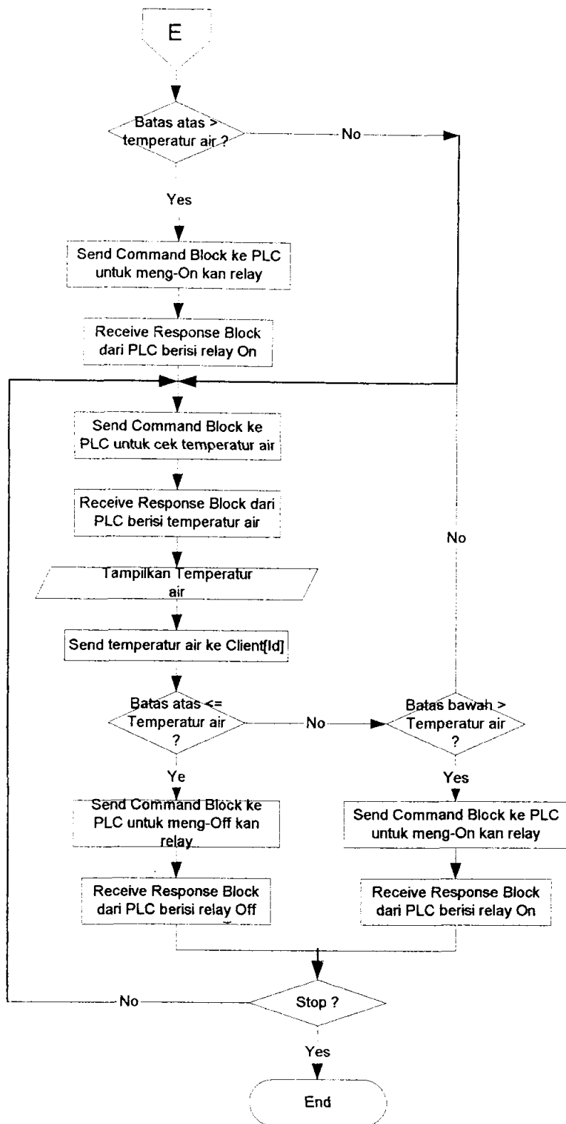
GAMBAR L-10 GAMBAR DIAGRAM ALUR LANJUTAN MENU APLIKASI (DIRECT CONTROL) SERVER DENGAN MEMANFAATKAN dWINSOCK
