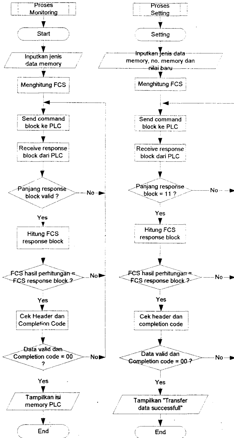
GAMBAR L-1 GAMBAR DIAGRAM ALUR MENU MONITORING DAN SETTING KOMPUTER-PLC
