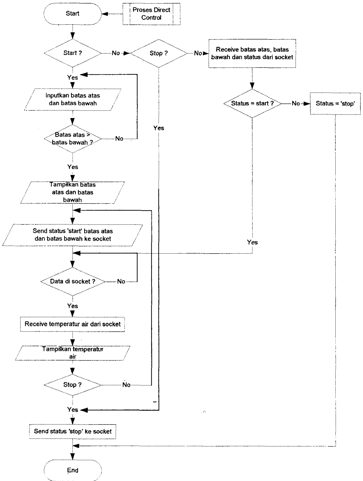
GAMBAR L-15 GAMBAR DIAGRAM ALUR MENU APLIKASI CLIENT (DIRECT CONTROL) DENGAN MEMANFAATKAN dWINSOCK
