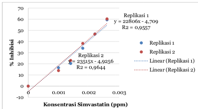
Gambar 2. Grafik konsentrasi simvastatin terhadap % inhibisi.
