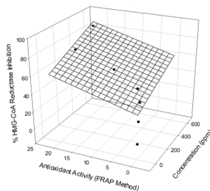
Gambar 7. Korelasi persentase penghambatan enzim HMGCo-A reductase dengan aktivitas antioksidan (metode FRAP).
