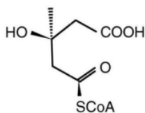
Gambar 5. Struktur HMG-CoA (Stancu and Sima, 2001).
