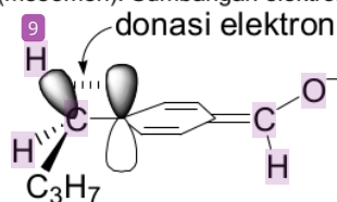
Gambar 3. Hiperkonjugasi
