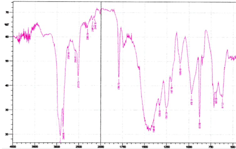
Gambar 2. Hasil identifikasi bahan paparan menggunakan FT-IR
