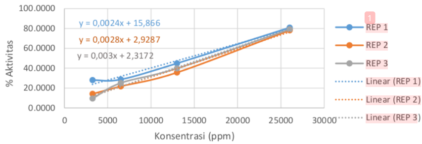
a. Senyawa (1a)
