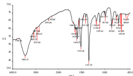
Gambar 3. Spektrum inframerah senyawa 4,4'-dinitrodibenzalaseton.
