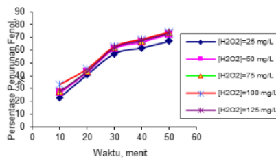
Gambar-3. Persentase Penurunan Konsentrasi Fenol akibat Oksidasi menggunakan reagen Fenton tanpa Radiasi UV
