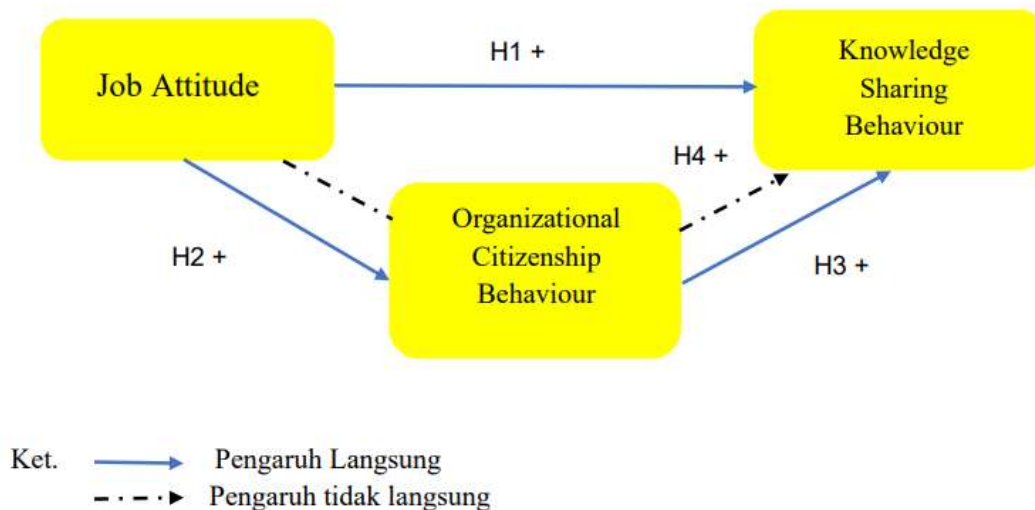
Gambar 1. Kerangka Penelitian
