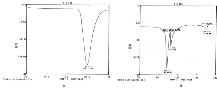
Gambar 2. Pola termogram DSC: (a) ibuprofen; (b) natrium ibuprofen hasil sintesis.
