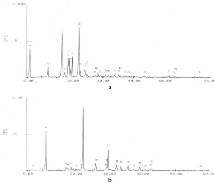
Gambar 5. Pola difraksi sinar-X: (a) ibuprofen; (b) natrium ibuprofen hasil sintesis.
