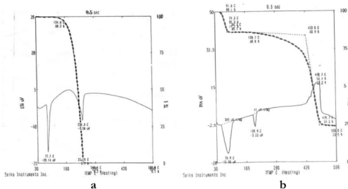
Gambar 1. Pola termogram TGA (garis putus-putus)/DTA (garis penuh): (a) ibuprofen; (b) natrium ibuprofen hasil sintesis.
