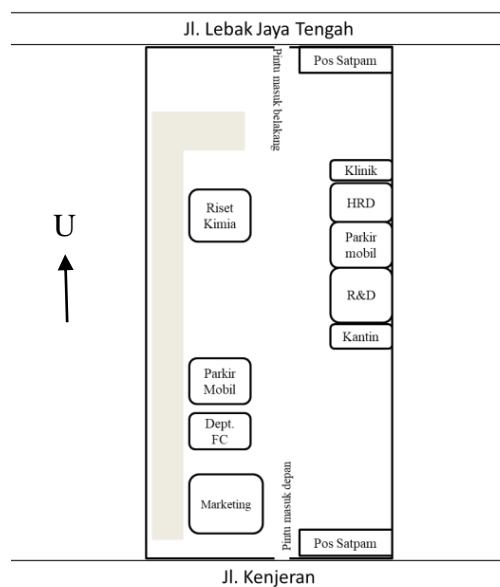
Gambar I.1. Tata letak pabrik
