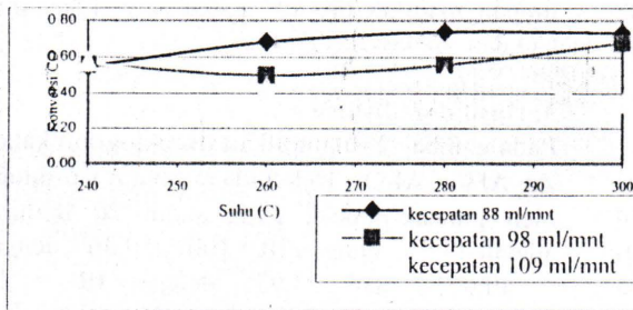
Gambar 3. Hubungan antara suhu terhadap konversi untuk katalis Cu-Zn-Al11/γ-Al 2 O 3 )
