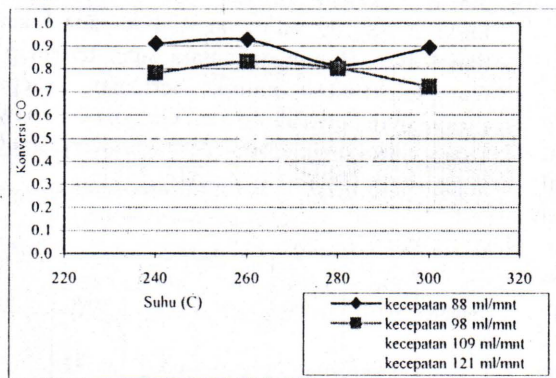
Gambar 4. Hubungan antara suhu terhadap konversi untuk katalis Cu-Zn-Al12/γ-Al 2 O 3
