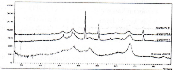
Gambar 2. Difraktogram Katalis-katalis Cu-Zn-Al/γ- Al 2 O 3 dengan IR = 33,21% dan 66,24° dengan IR = 15,36%. Selain itu keberadaan logam Al terdapat dalam bentuk Al 2 O 3 ditunjukkan oleh puncak pada sudut 2θ adalah 32,38° dengan IR = 26,22%; 39,01° dengan IR = 23,64%; 50,46° dengan IR = 40,02%; dan 66,24° dengan IR = 15,36%. Dari uji AAS tipe ICPS (Inductively Coupled Plasma Spectrometer), katalis ini memiliki persen loading Cu = 9,49%; Zn = 2,70% dan Al = 4,42%. Untuk katalis lainnya persen loading logam-logam ditabelkan pada Tabel 4.
