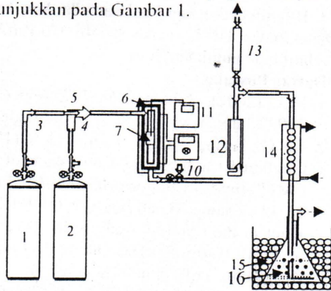
Gambar 1. Rangkaian Alat Konversi Syngas Menjadi DME Keterangan Gambar
